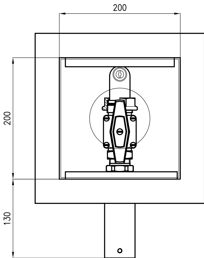
PE D32 SDR11
