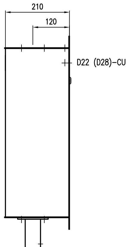
Védőcsőtartó hüvelyezés (PE-acél összekötő szerelésekor ideiglenesen kivethető)
