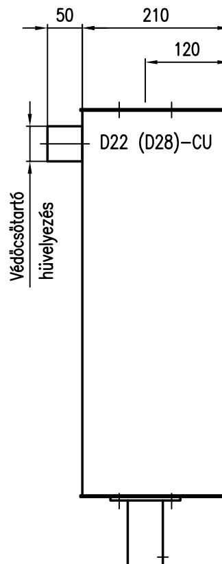
Védőcsőtartó hüvelyezés
