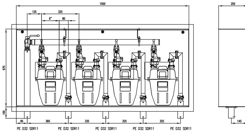
Beépíthető szabályozó: 4db KMS-1-25A típusú gázmérő nyomásszabályozó (a mérő kilepő oldalán KMS közdarabbal) Az alapkitelű berendezés további tartozékai: 5db D32 méretű, hajított acél védőcsővezetés
